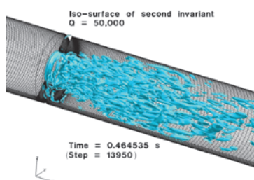
図1. オリフィス下流の渦構造の数値シミュレーション
